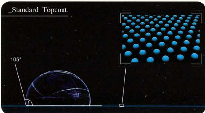
Standard AR
